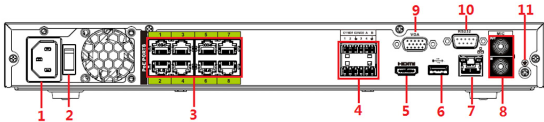
Abbildung 2-7 NVR4216-16P-I
