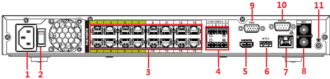
Abbildung 2-6 NVR5216-8P-I
